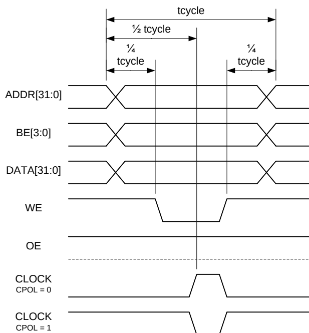
Рисунок 34. Диаграмма записи
