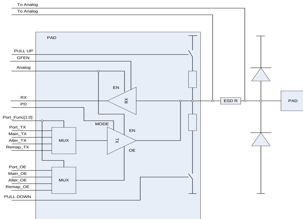
Рисунок 32. Порты ввода-вывода
