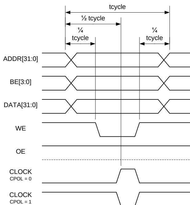
Рисунок 38. Диаграмма записи
