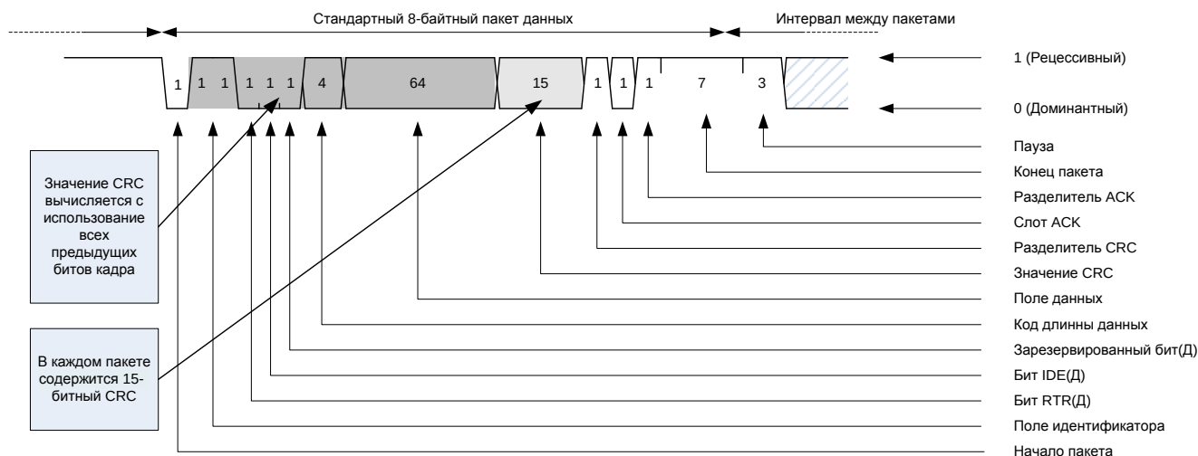
Рисунок 58. Контроль CRC
