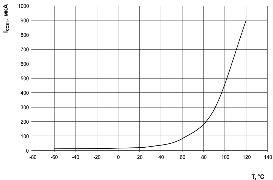
Рисунок 138. Зависимость статического тока потребления в режиме покоя (регулятор напряжения включен) от температуры
