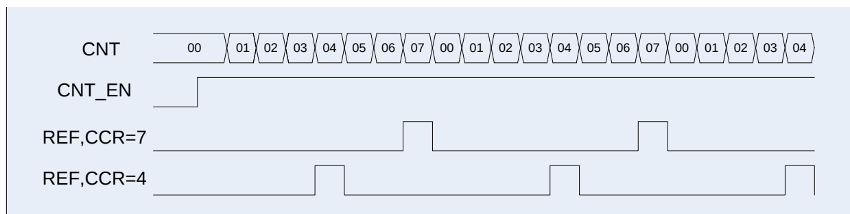
Рисунок 83. Диаграмма работы схемы в режиме ШИМ, CCR1_EN=0
