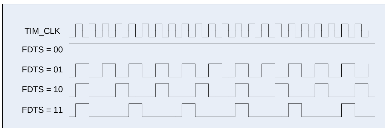
Рисунок 74. Диаграммы возможных частот семплирования данных (FDTS)
