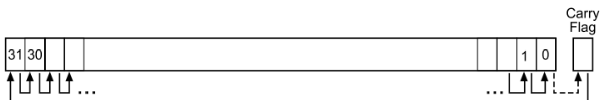
Рисунок 26. Инструкция RRX
