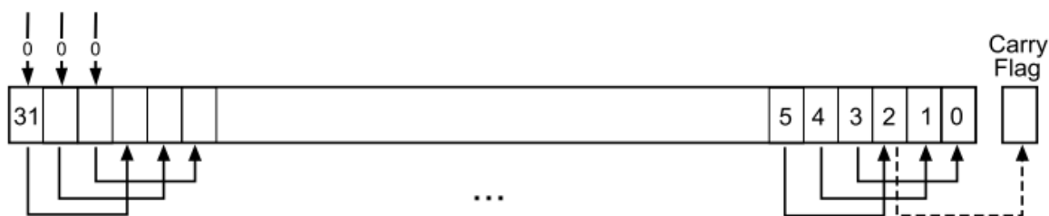
Рисунок 23. Инструкция LSR # 3
