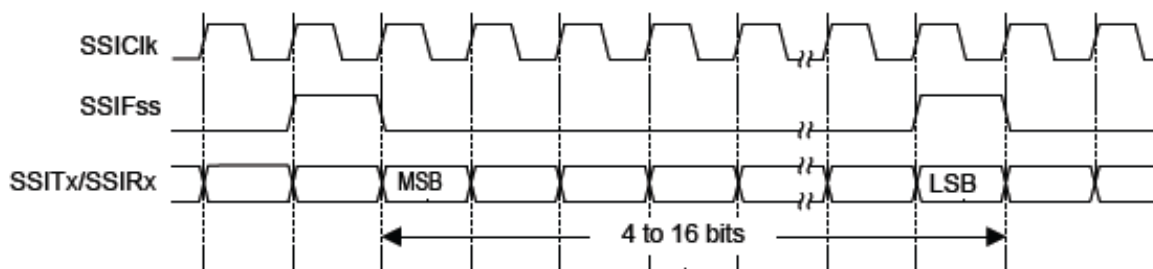
Рисунок 100. Формат синхронного обмена протокола SSI (непрерывный обмен)
