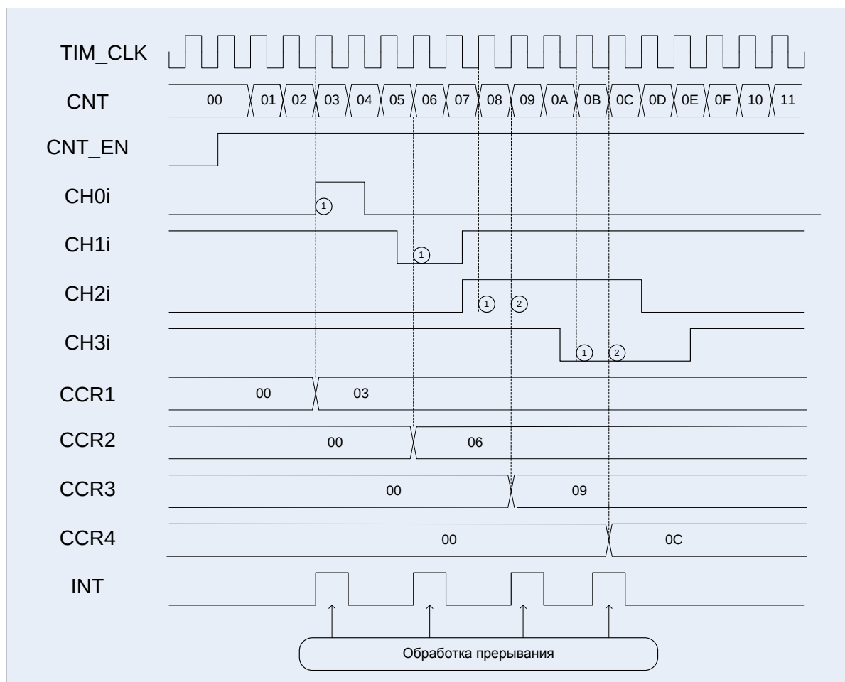
Рисунок 89. Диаграммы примера работы в режиме захвата
