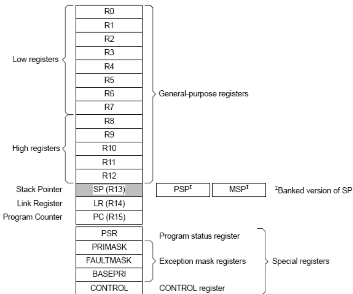
Рисунок 21. Регистры ядра
