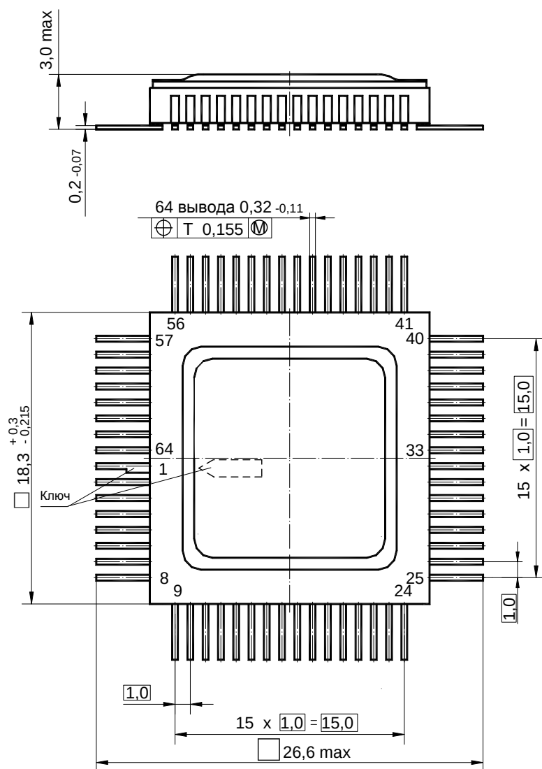
Рисунок 143. Корпус N18.64-1B
