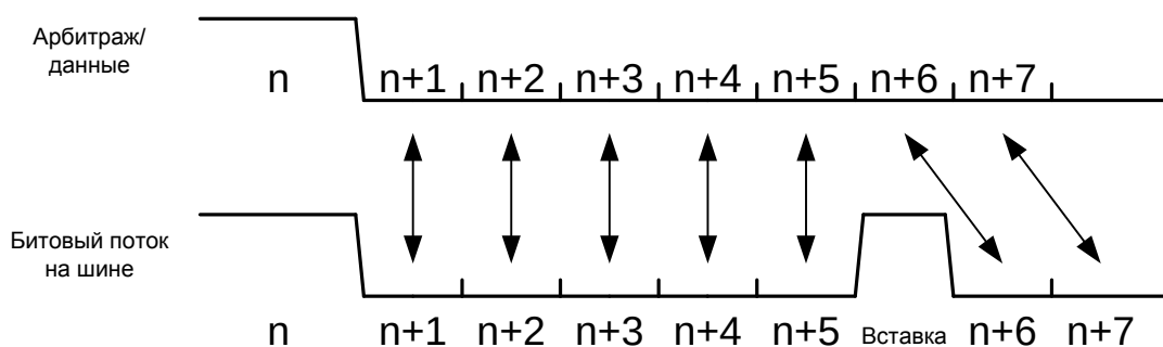
Рисунок 60. Битстаффинг
