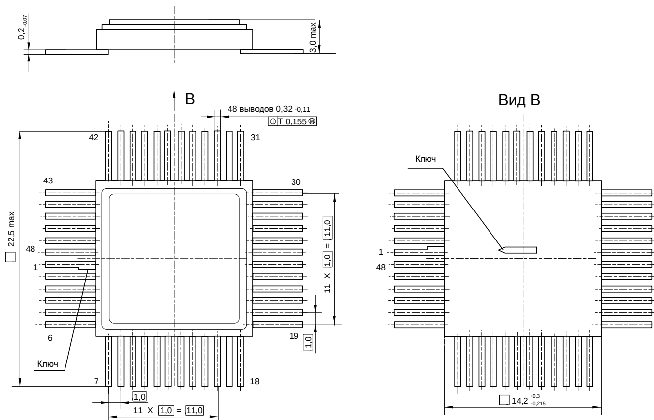
Рисунок 144. Корпус Н16.48-1В
