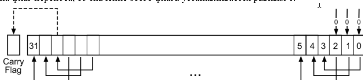
Рисунок 24. Инструкция LSL # 3
