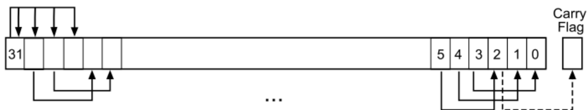
Рисунок 22. Инструкция ASR # 3
