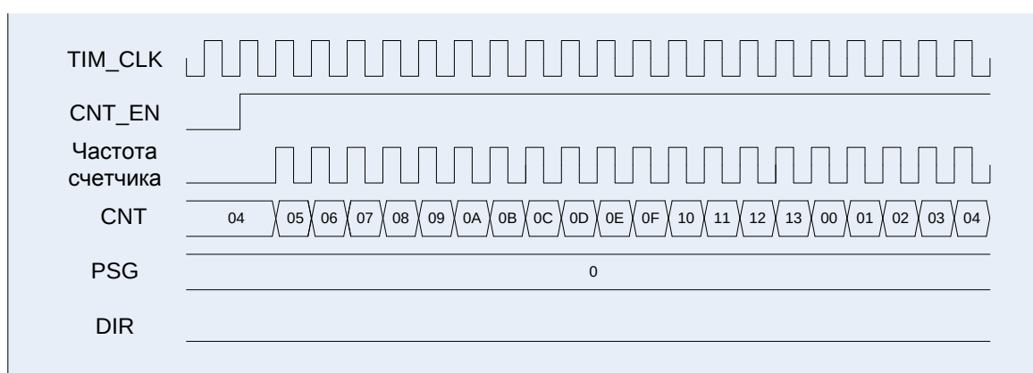
Рисунок 64. Диаграммы работы таймера, счет вверх
