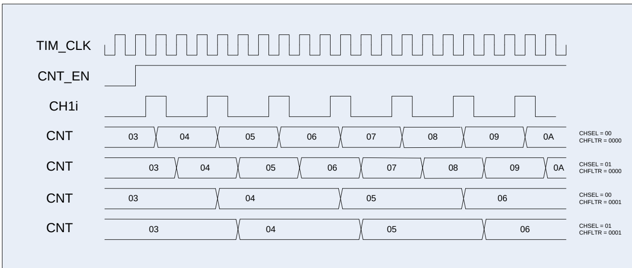
Рисунок 76. Диаграмма внешнего тактирования с разными вариантами фильтра
