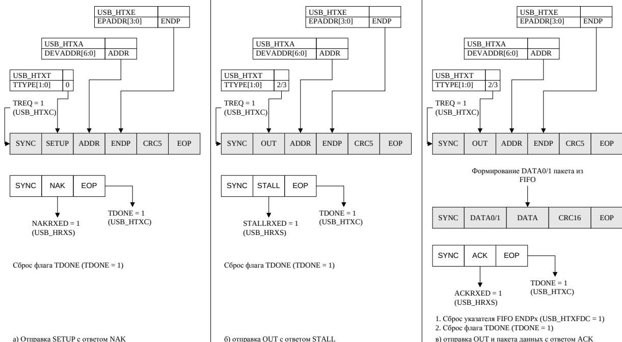
Рисунок 43 (а, б, в). Транзакция SETUP/OUT (USB Host)
