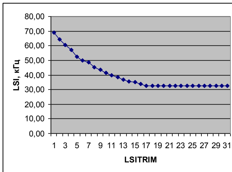
Рисунок 30. Зависимость частоты LSI от значения LSITRIM
